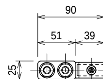
Z端子 片側付 (品番 : S7141)
