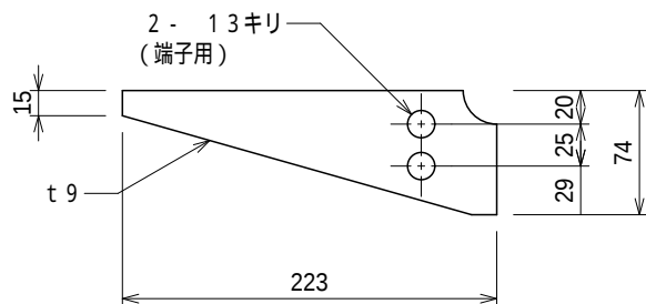
架台リブ詳細図 (端子取付部) S = 1 : 4
