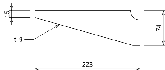
架台リブ詳細図 S = 1 : 4
