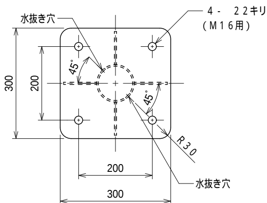
架台詳細図
