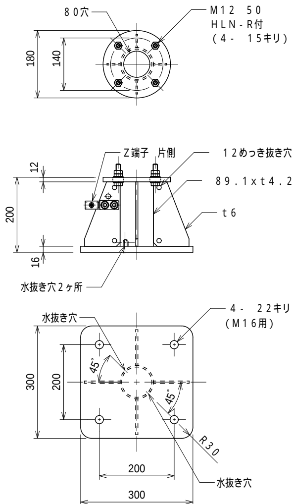
架台詳細図
