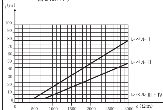
図2 保護レベルに応じた接地極の最小長さ l_1 レベルⅢ・Ⅳは大地抵抗率 \rho (ロー) と無関係である。
