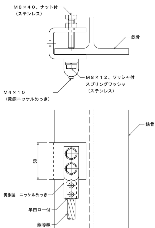
接続クランプ
