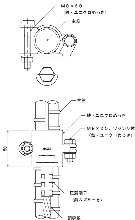
接続クランプ
