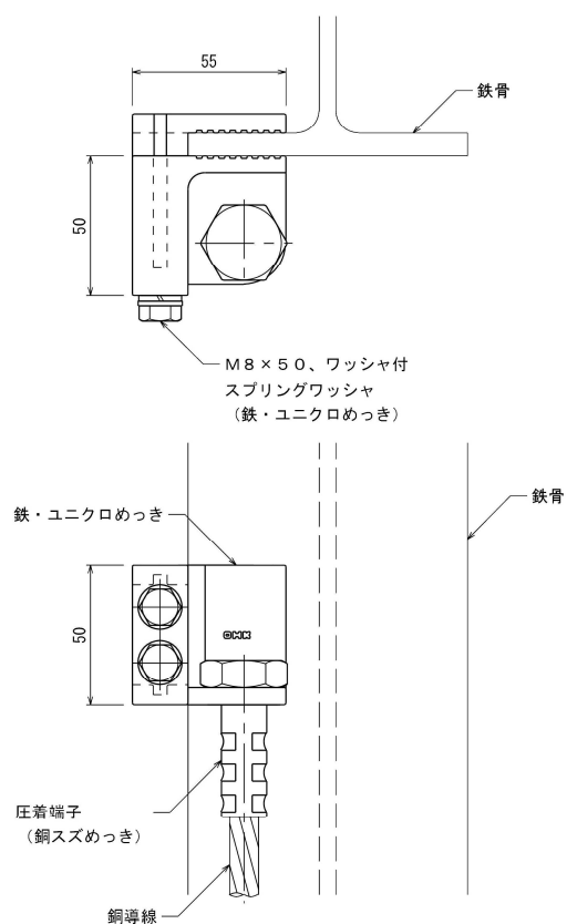
鉄骨接続端子
