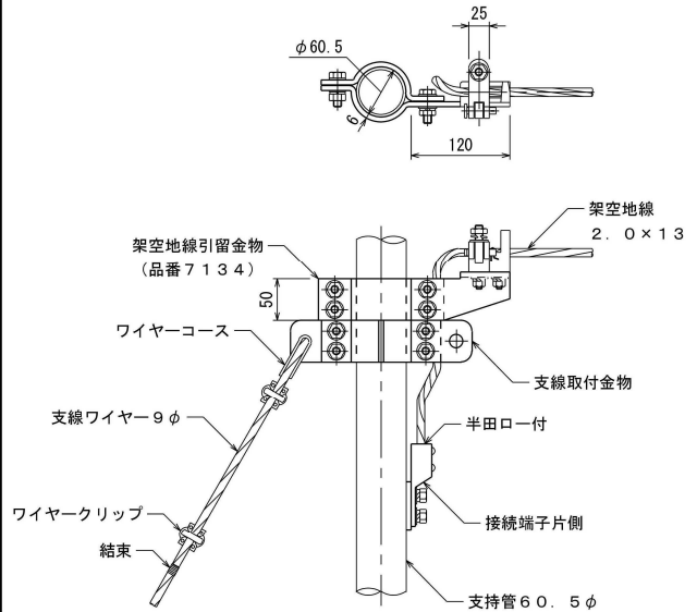
品番 7 1 3 4 架空地線引留金物 直角用
