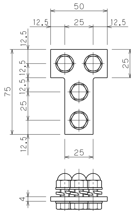
品番 7513 T型継手
