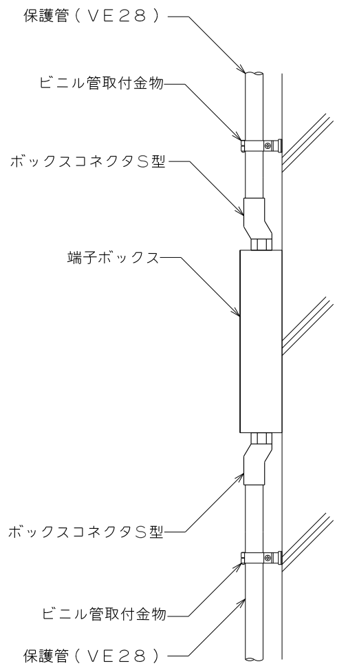
施工参考図
